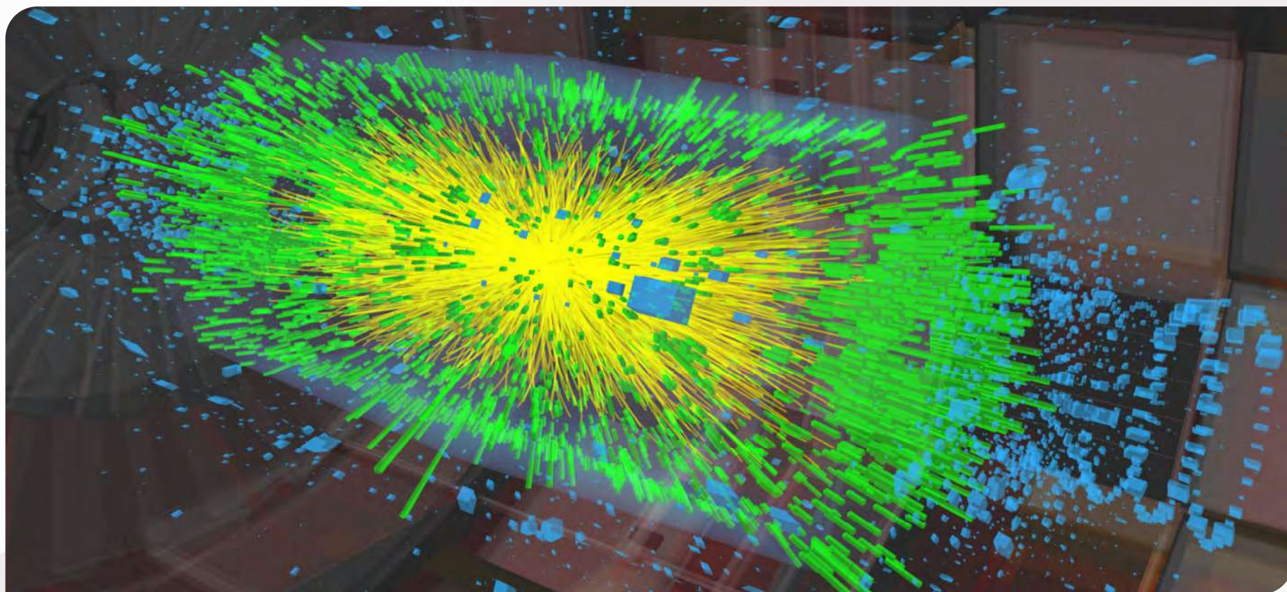
Evento de colisión de iones pesados registrado por el detector CMS en el LHC en septiembre de 2023. Las trayectorias reconstruidas de miles de partículas revelan la extraordinaria densidad de materia creada en estas colisiones, que permiten estudiar el plasma de quarks y gluones. Imagen: CERN / Colaboración CMS.
