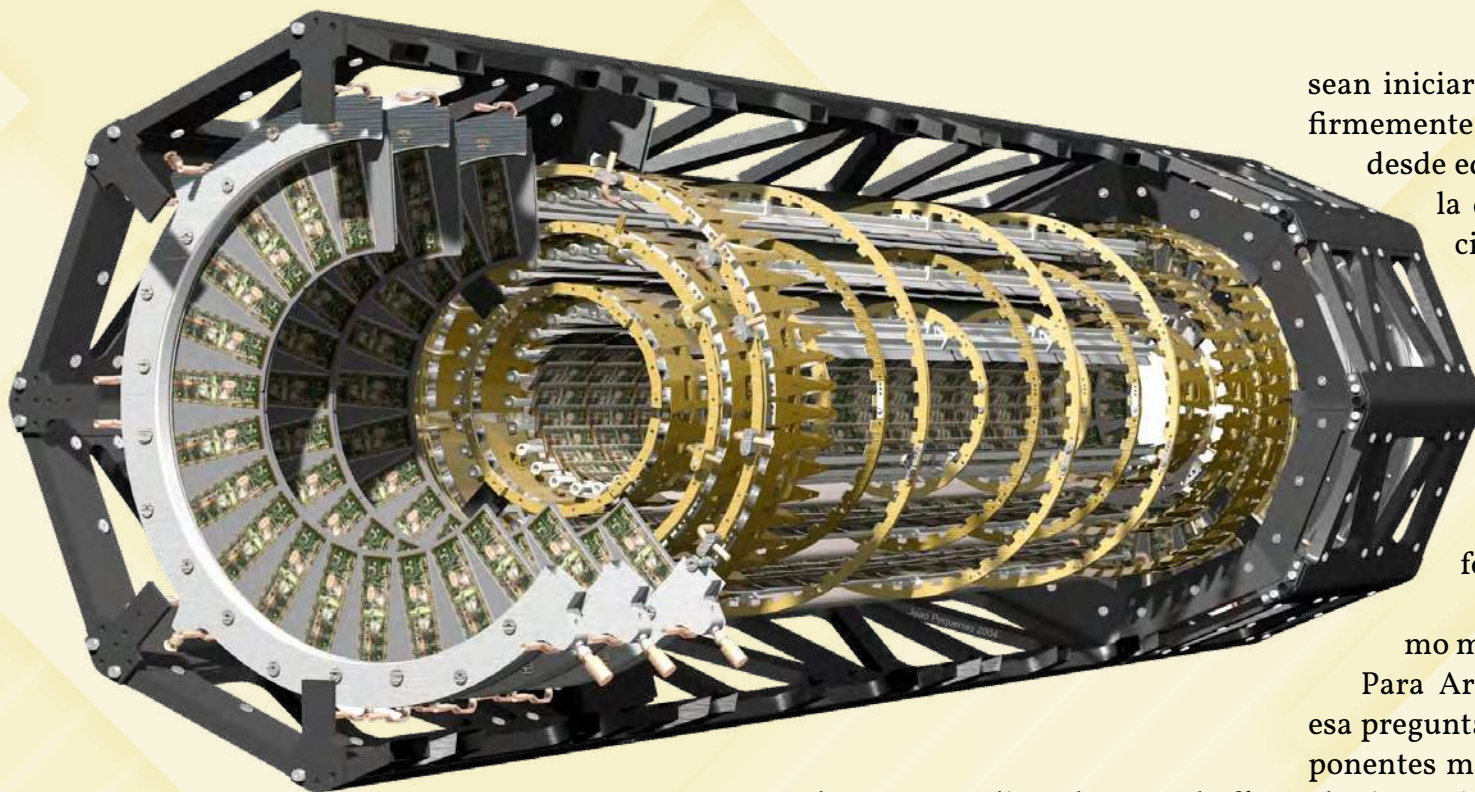
Imagen generada por computadora del detector de píxeles, la capa más interna del detector ATLAS, que registra la trayectoria de las partículas producidas en las colisiones.
