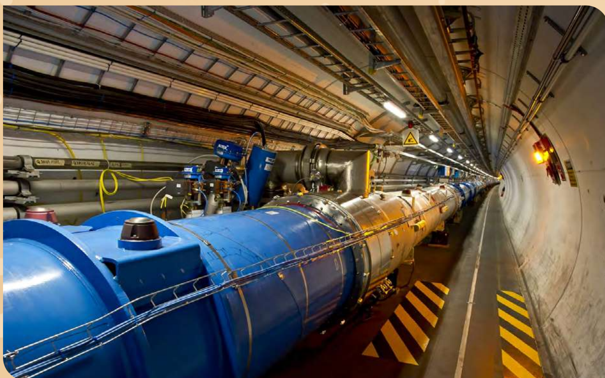
El túnel del Gran Colisionador de Hadrones (LHC) del CERN. Sus imanes superconductores guían haces de protones a energías cientos de millones de veces mayores que las alcanzadas en los primeros tubos de rayos catódicos. Foto: CERN.
