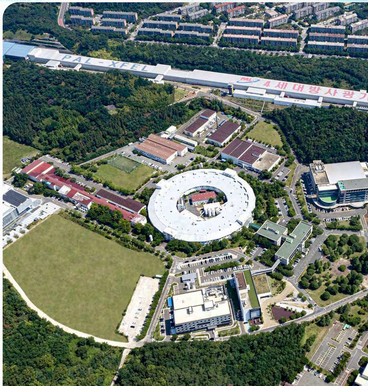
Pohang Light Source es el sincrotrón de Corea del Sur, activo desde 1995. Foto: Pohang Accelerator Laboratory (PAL).
