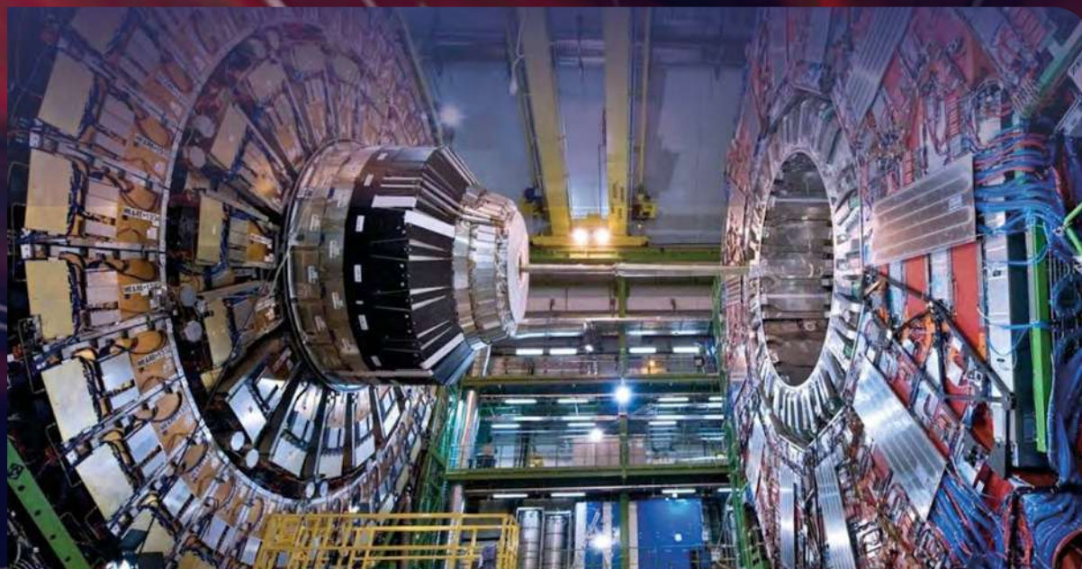
El Gran Colisionador de Hadrones -LHC- es el acelerador de partículas más grande y potente que ha existido. Se encuentra en la frontera francosuiiza cerca de Ginebra. Foto: CERN / Colaboración ATLAS.
