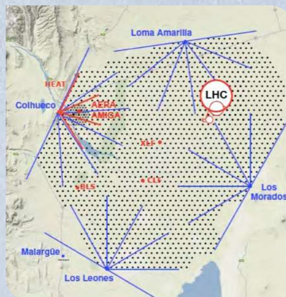
Mapa del Observatorio comparado con el LHC. Imagen: Colaboración Pierre Auger.
