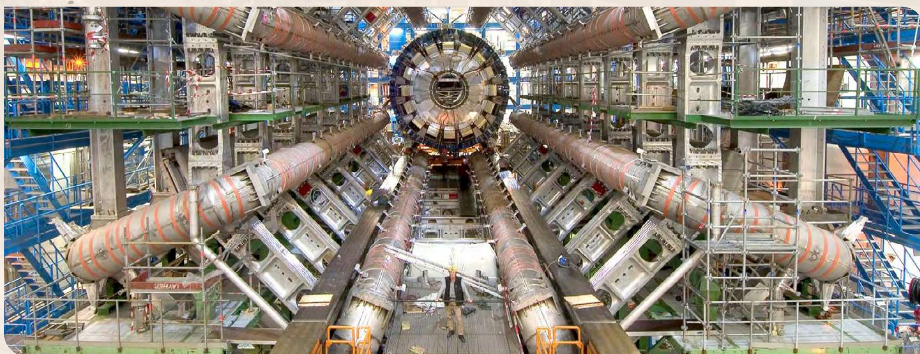
Interior del detector ATLAS durante su construcción en el CERN. La persona en el centro permite apreciar la escala de uno de los instrumentos científicos más grandes jamás construidos. Foto: CERN / Colaboración ATLAS.
