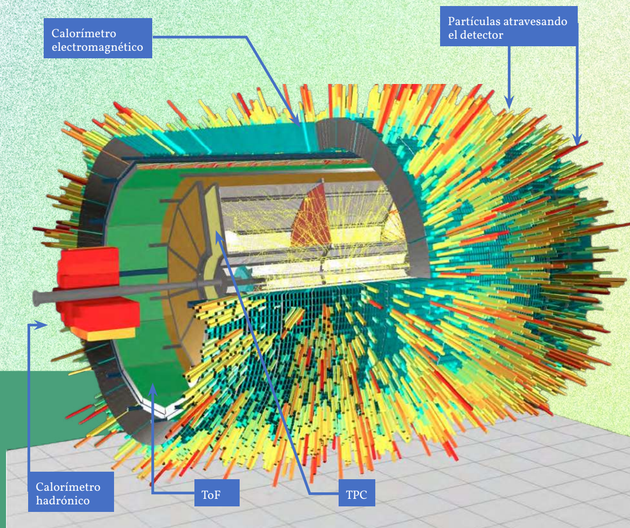
Simulación de partículas producidas en una colisión de iones pesados, atravesando los diferentes sistemas del MPD.
